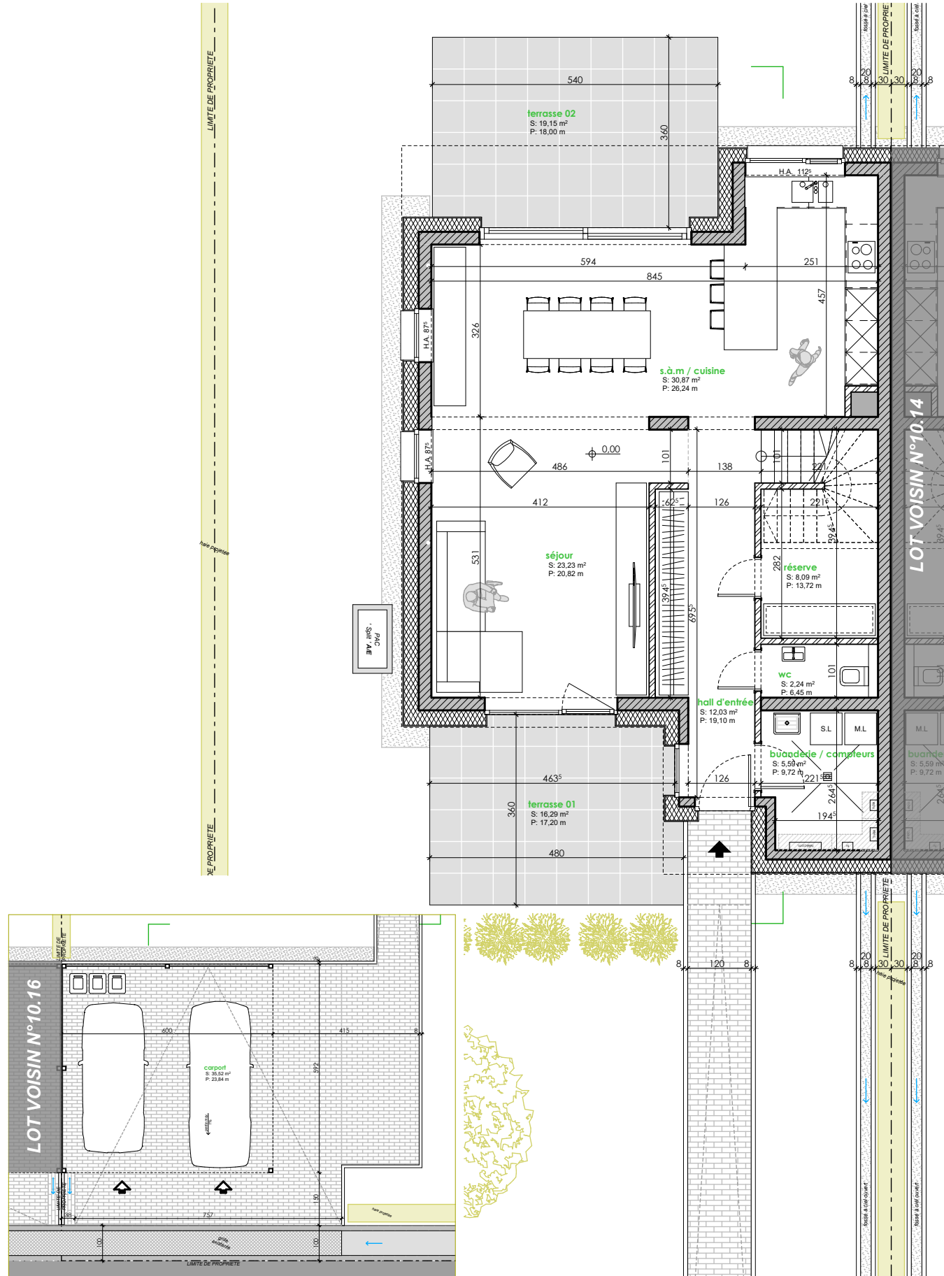
Rez-de-chaussée (carport) éch. 1/150
