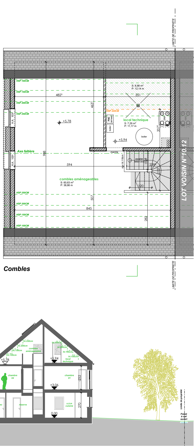
Coupe de principe éch. 1/200
