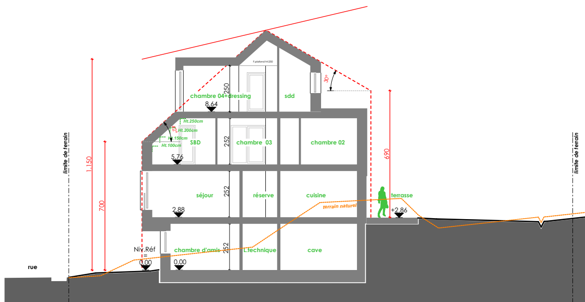
Coupes A-A
