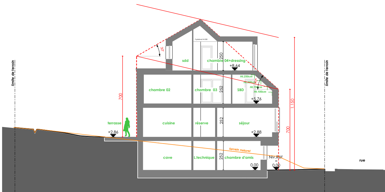
Coupes A-A
